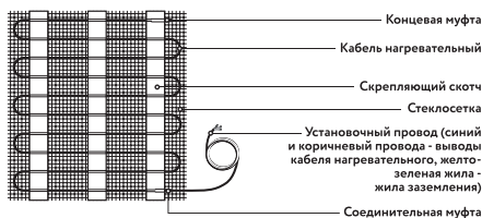
Рис. 1. Конструкция мата
