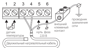
Рис. 2. Схема подключения мата к электрической сети
